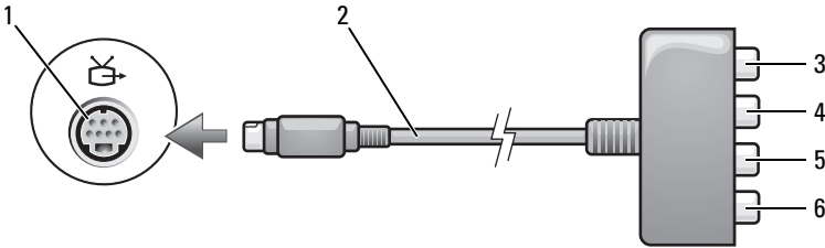
1 S-video TV-out 커넥터 2 복합 비디오 어댑터 3 S/PDIF 디지털 오디오 커넥터 4 Pr( 빨간색 ) 구성요소 비디오 출력 커넥터 5 Pb( 청색 ) 구성요소 비디오 출력 커넥터 6 Y( 녹색 ) 구성요소 비디오 출력 커넥터
